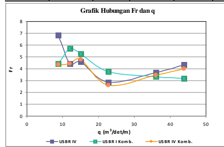
Gambar 8b. Hubungan antara Fr dan q diakhir saluran peluncur.(section 14)
